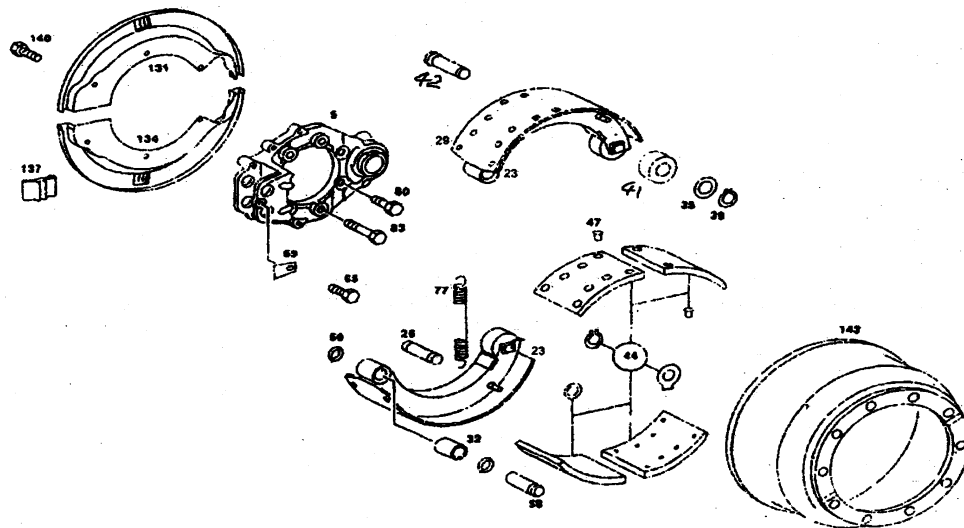
卡车后桥总成Rear axle assembly
