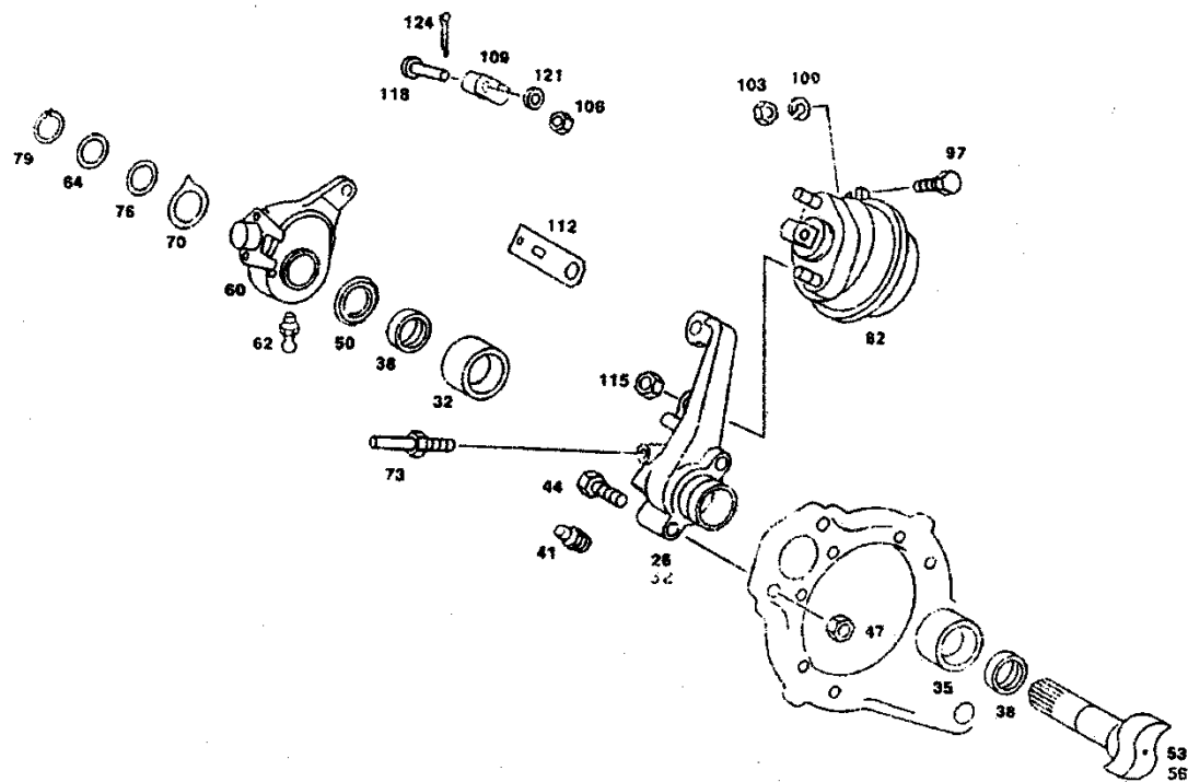
非驱动前桥总成 Front axle assembly
