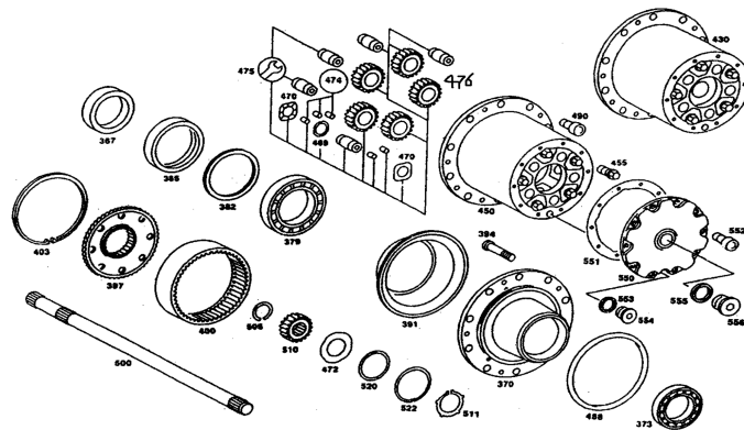
卡车后桥总成Rear axle assembly
